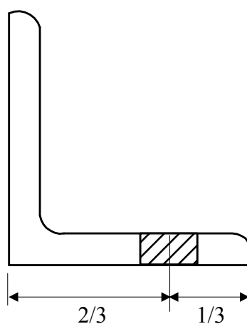
Angles
